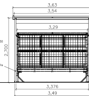
SEZIONE ESSICCATOIO
