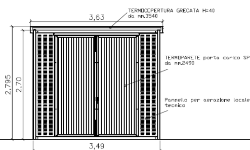
VISTA (A) porta locale tecnico
