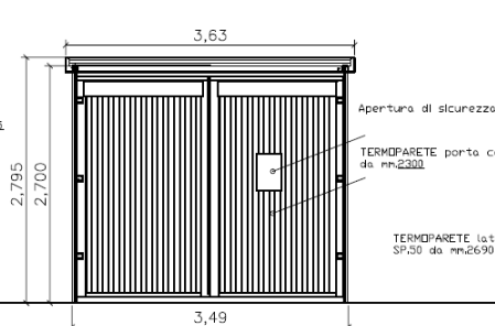
VISTA (B) porta di carico
