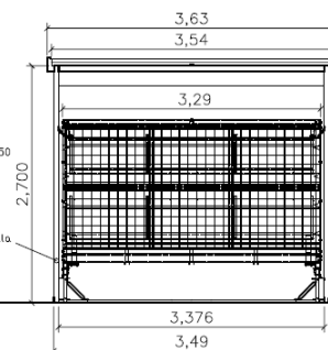
SEZIONE ESSICCATOIO
