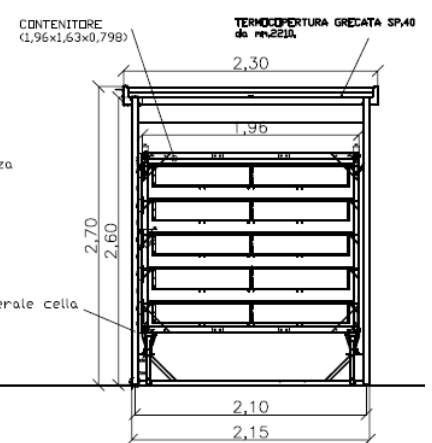
SEZIONE ESSICCATOIO
