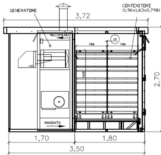
VISTA LATERALE
